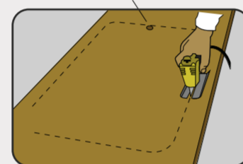
Furo Ø 10 mm para iniciar o corte com a serra tico tico Agujero de Ø 10 mm para comenzar el corte con la sierra caladora Hole Ø 3/8" for starting with jigsaw
