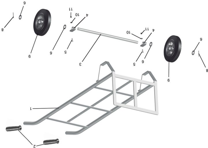
Vista explodida | Detailed drawing | Dibujo desglóce
