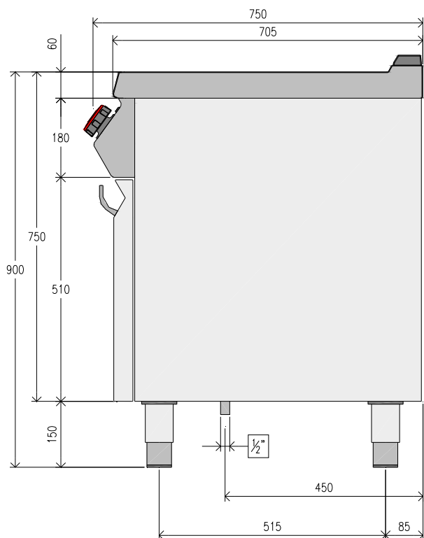
Vista lateral
