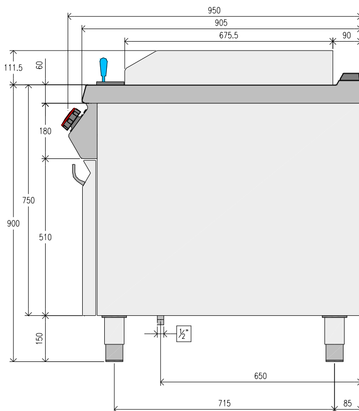
Vista lateral
