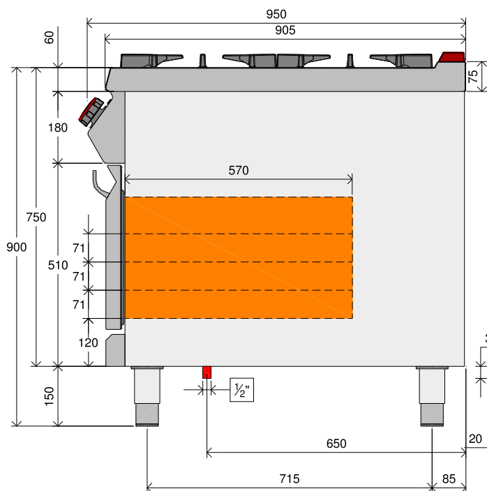
Vista lateral
