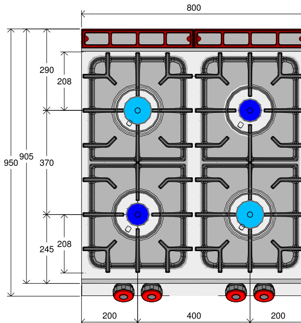
Vista superior
