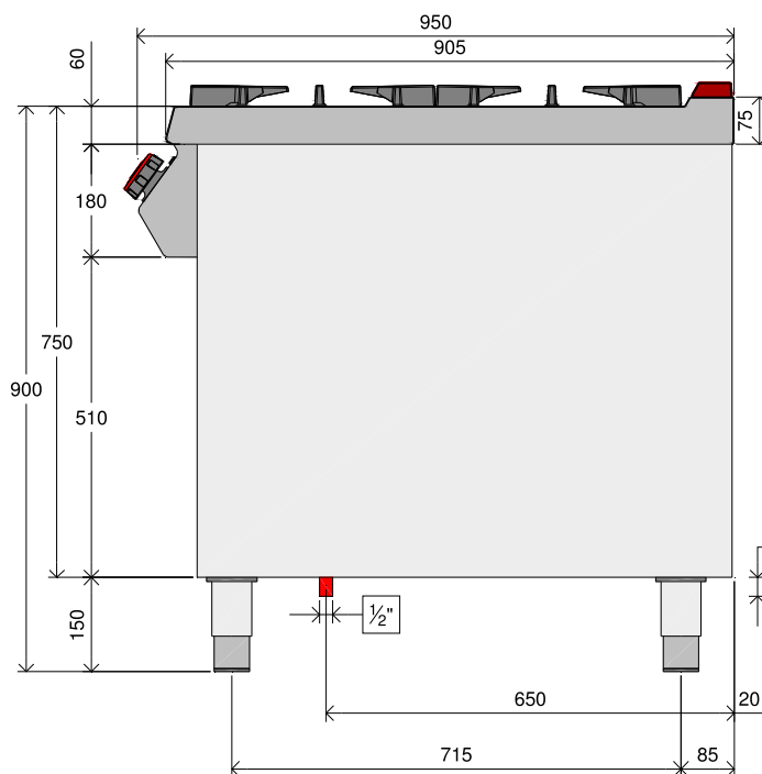
Vista lateral
